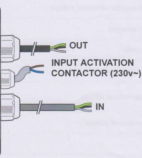
EN - Wiring connections
