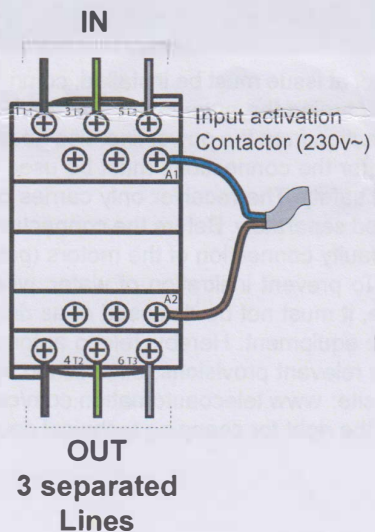
EN - Wiring connections
