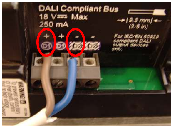
GRAFIK Eye:OUTPUT SIGNAL DALI
